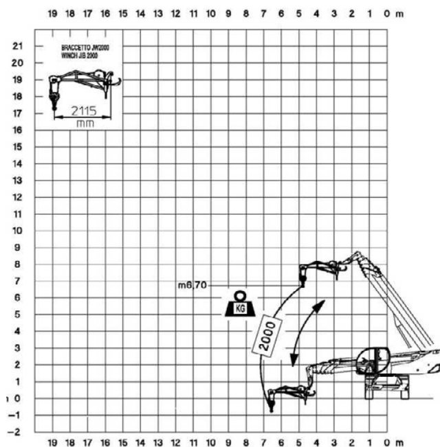
Braccetto JW 2000 laterale su ruote
