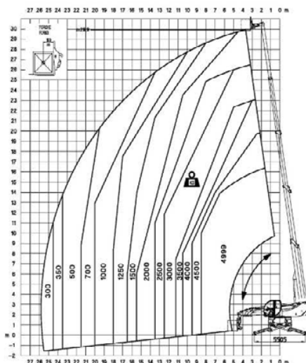
Gancio 5 T su stabilizzatori
