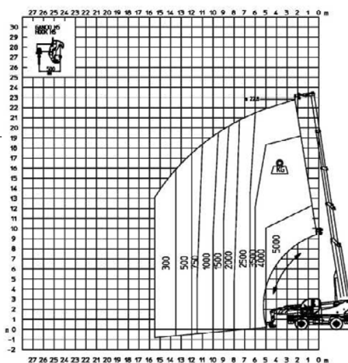
Argano 5 t frontale su gomma
