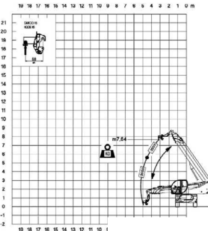
Argano 5 t laterale su gomma
