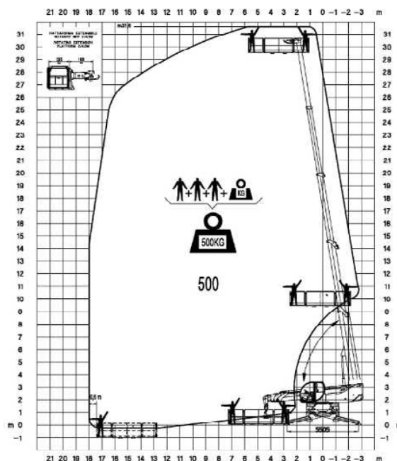
Piattaforma estensibile rotante REP 2/5
