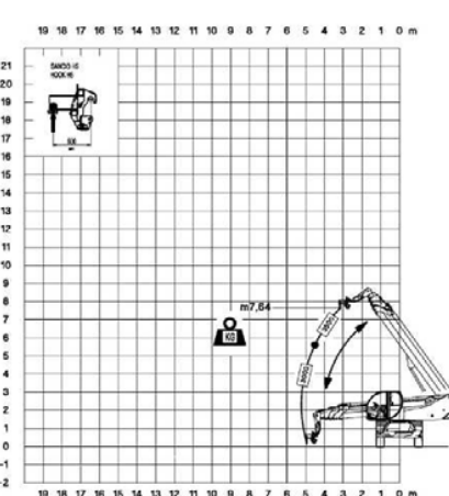
Gancio 5 T laterale su ruota
