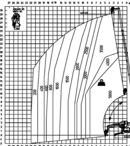
Argano 5 t su stabilizzatori
