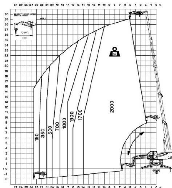
Piattaforma estensibile rotante REP 2/5
