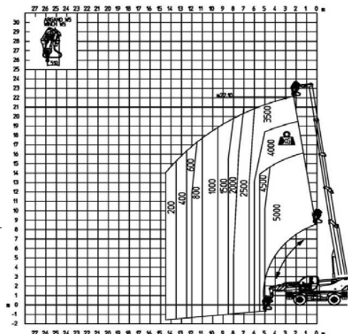
Argano 5 t frontale su gomma
