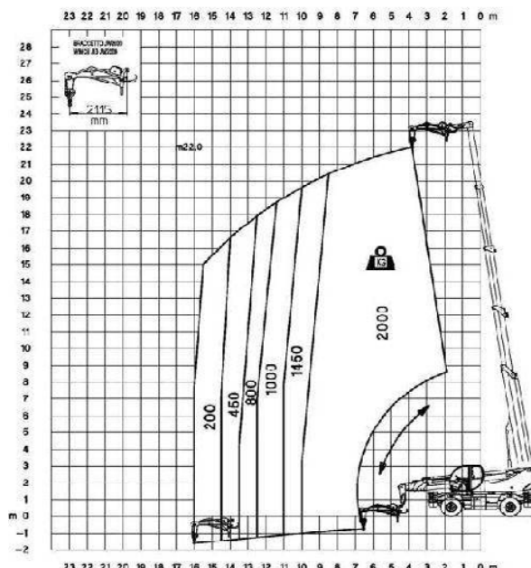
Braccetto JW 2000 laterale su ruote
