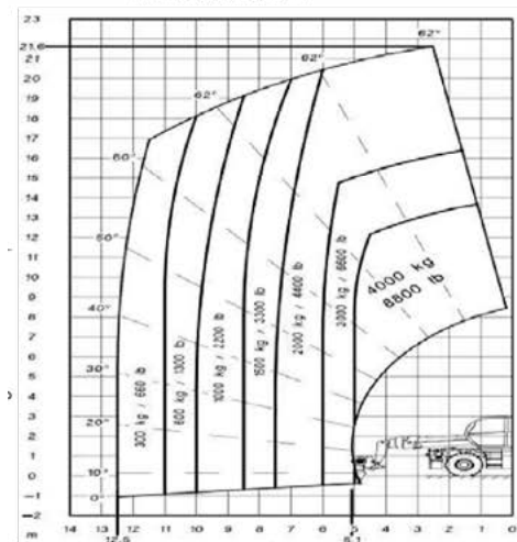
BRACCETTO P 600 FRONTALE SU RUOTE
