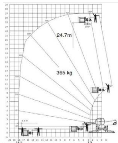
ROTAZIONE CESTA SU STABILIZZATORI
