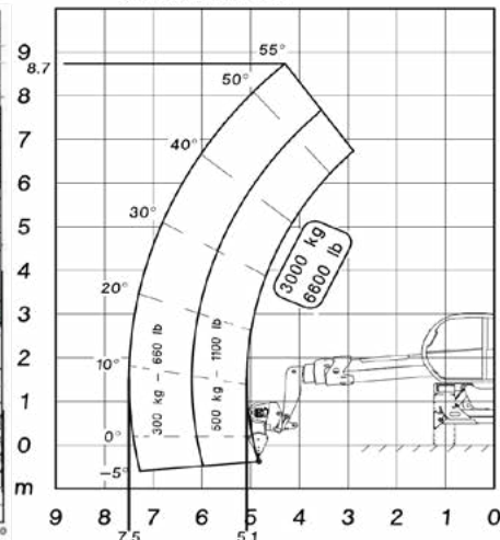
BRACCETTO P 600 LATERALE SU RUOTA
