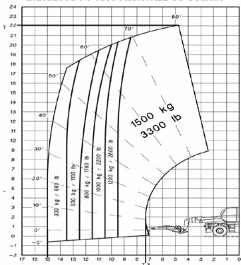
BRACCETTO PT 1500 FRONTALE SU GOMMA
