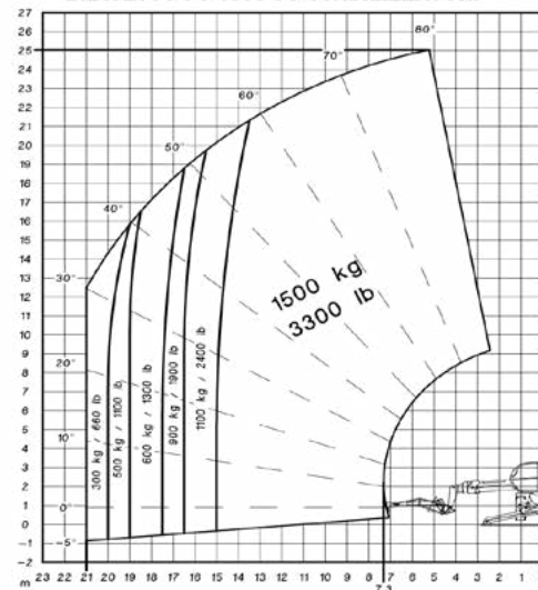
BRACCETTO PT 1500 SU STABILIZZATORI
