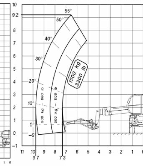
BRACCETTO PT 1500 LATERALE SU GOMMA
