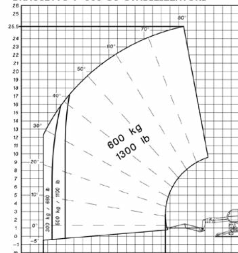
BRACCETTO P 600 SU STABILIZZATORI
