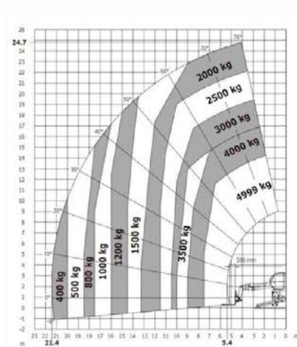
GANCIO PC 40 SU STABILIZZATORI
